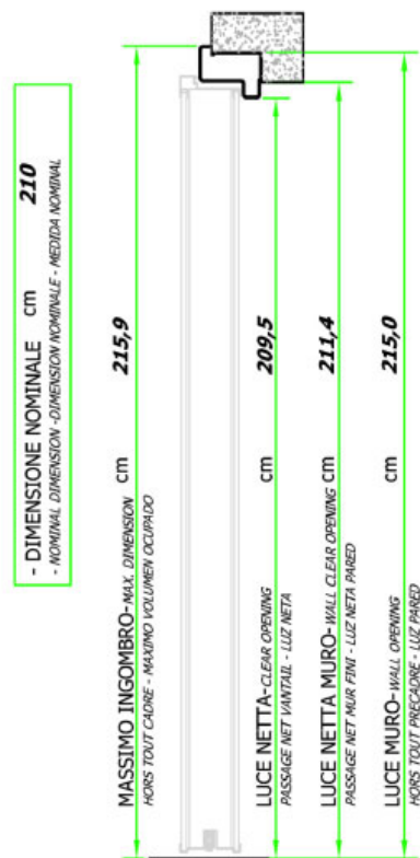
SEZIONE VERTICALE
