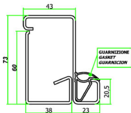
ACCOPPIAMENTO FALSO-TELAIO
