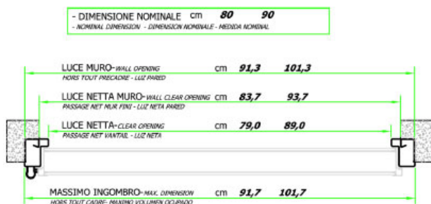
SEZIONE ORIZZONTALE
