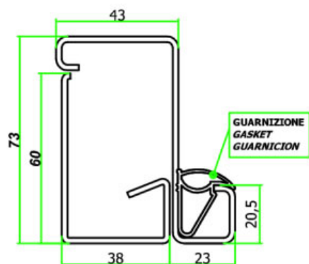
ACCOPPIAMENTO FALSO-TELAIO
