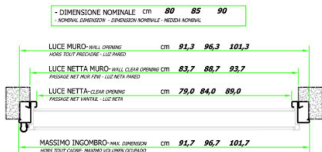
SEZIONE ORIZZONTALE
