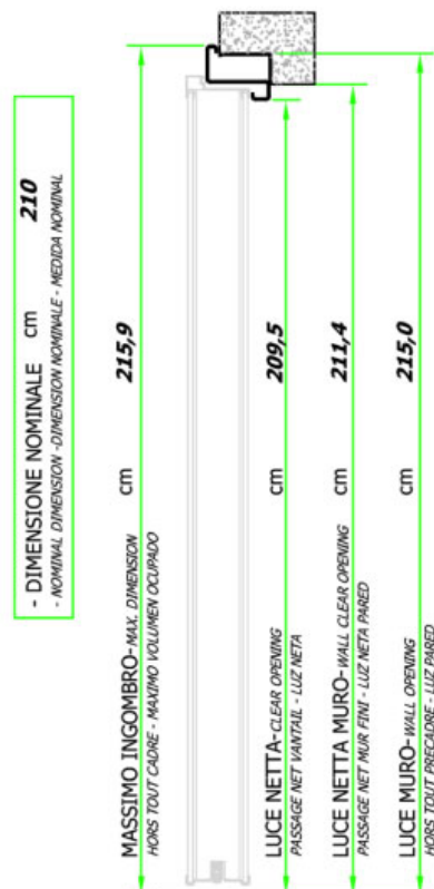
SEZIONE VERTICALE
