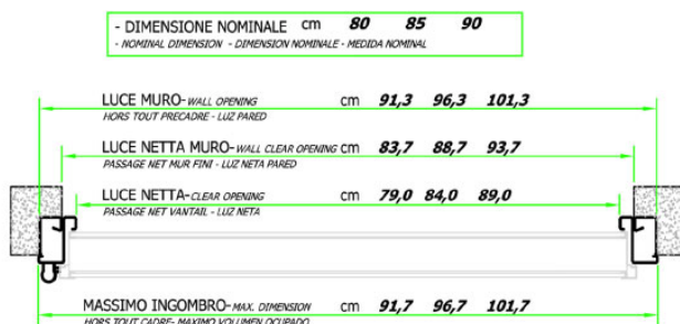
SEZIONE ORIZZONTALE
