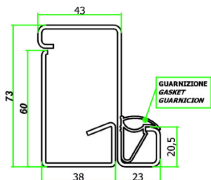
ACCOPPIAMENTO FALSO-TELAIO
